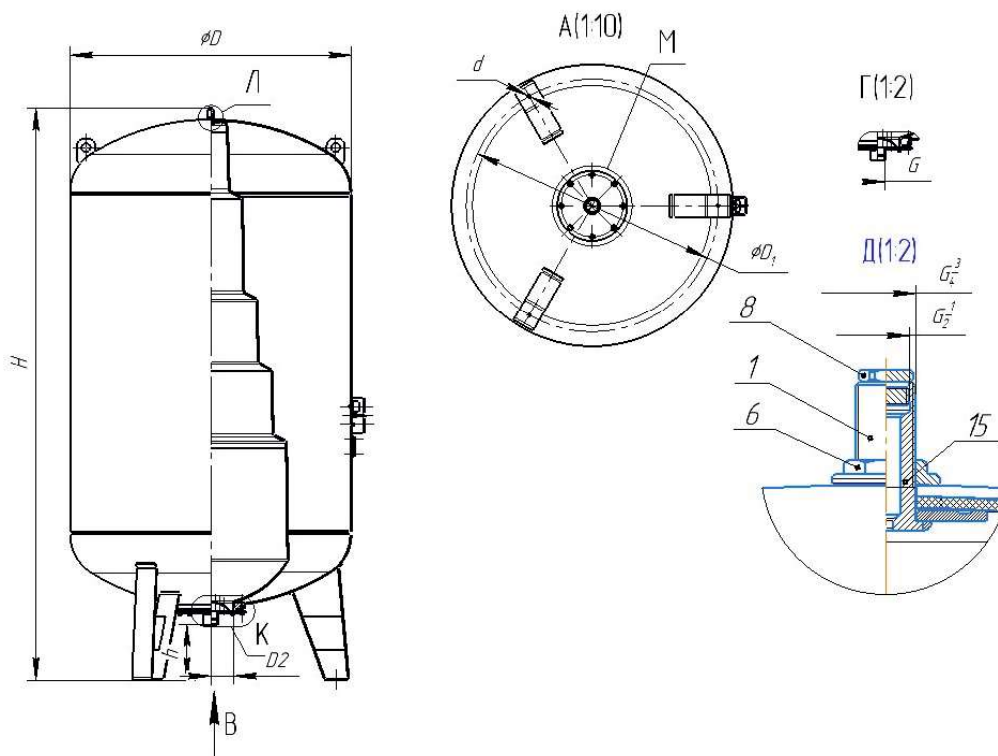
Модель WAV 1500-3000
